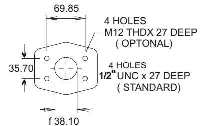
1-1/2" SAE FLANGE
