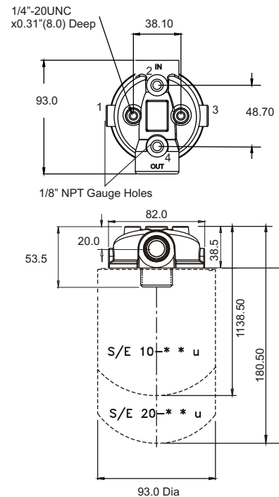
IF*4-06N-10-**-U Wt 0.85kg IF*4-06N-20-**-U Wt 1.05kg
